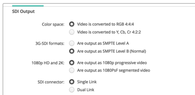
У цій секції можна налаштувати виведення SDI-відео
