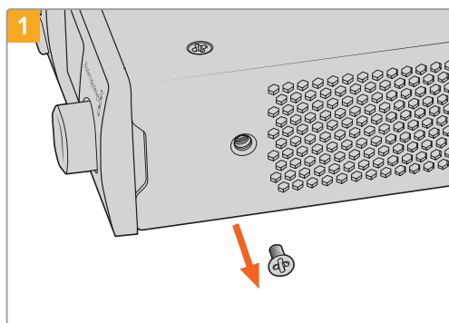
Entfernen Sie die 5mm-M3-Schraube nahe der Frontblende
