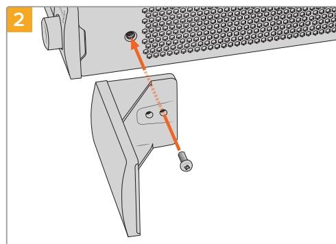
ブランクパネルをネジ穴に揃え、同梱のM3 (9mm) ネジで固定します。
