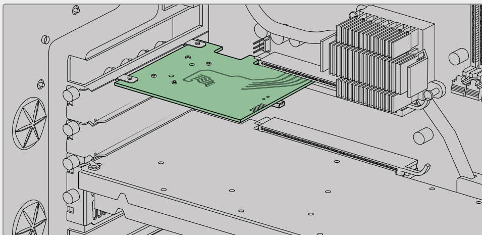
Karta PCIe jest włożona do gniazda PCIe Gen 2 w komputerze.
