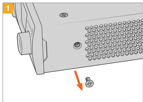
フロントの前面近くにあるM3 (5mm) 皿頭ネジを取り除きます。
