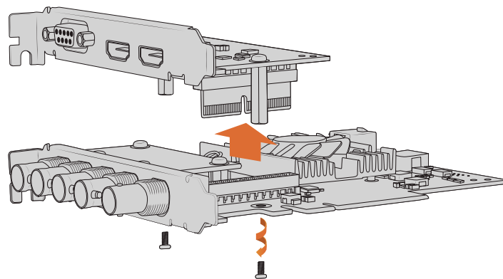
메자닌 카드는 쉽게 제거 및 설치할 수 있습니다.
